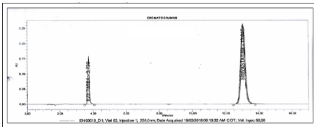
Figura N°4. Cromatograma de la solución muestra.
